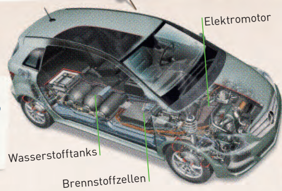
Abbildung 5: Querschnitt eines Wasserstoffautos
